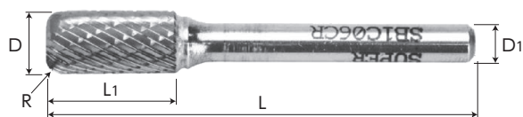
コーナーR刃
