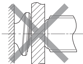
カムが傾いた状態での取付けは禁止
