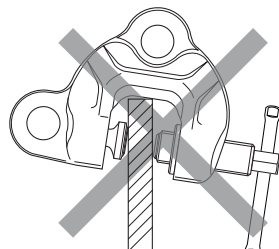
本体が傾いた状態での取付けは禁止
