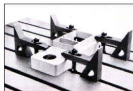
ステップクランプとステップブロックの組合せ
