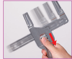
■クイックウォーム機構
