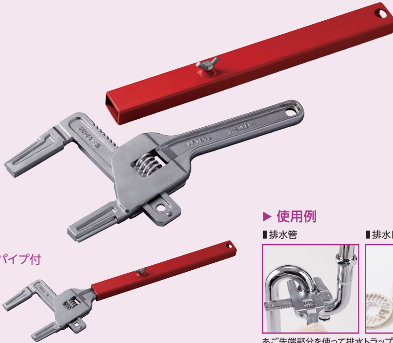
■クイックウォーム機構
