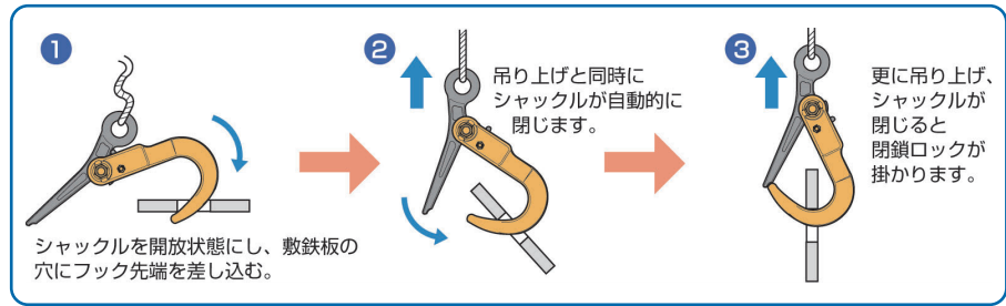
■敷鉄板吊り上げ時の操作方法
