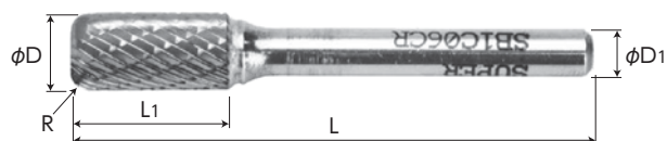
コーナーR刃
