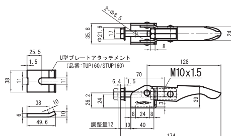
TLA160F/STLA160F
