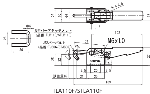
TLA110F/STLA110F
