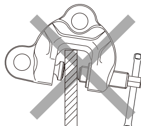
本体が傾いた状態での 取り付けは禁止
