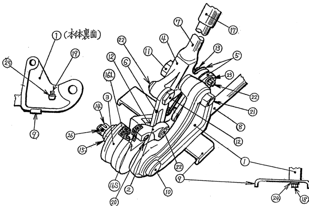
NK3W 部品表
