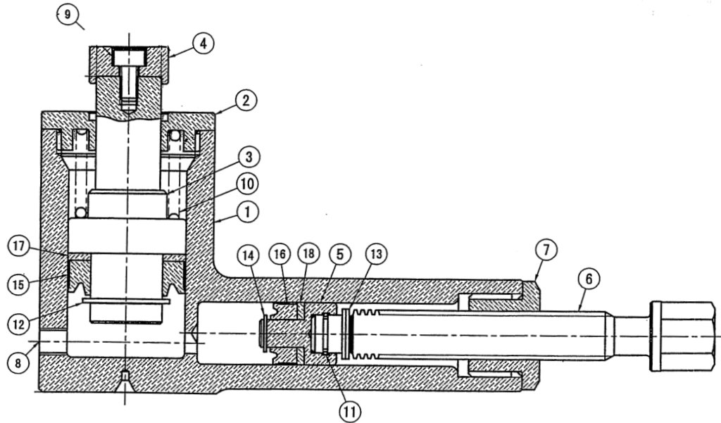
SW8N・16N 部品表
