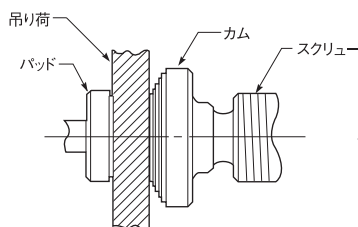
正しい取付状態
