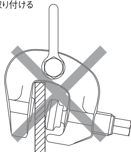
本体が傾いた状態での 取り付けは禁止
