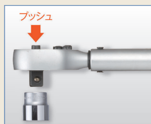
ソケットホールド機構
