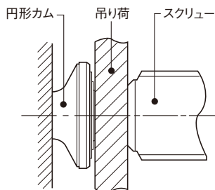
正しい取付状態
